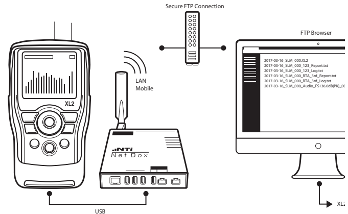
Lärm-Messtation mit FTP-Fernabfrage
