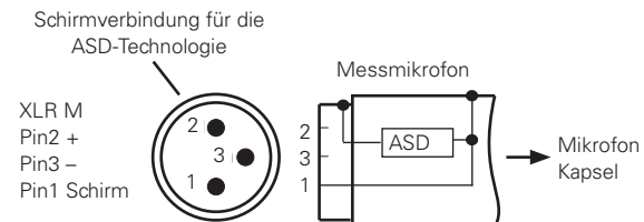
Verbindungsdiagramm der Messmikrofone mit elektronischem Datenblatt
