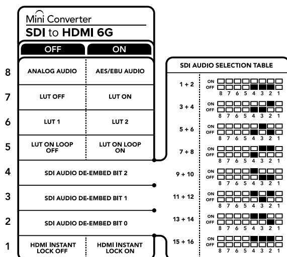
El diagrama situado en la parte inferior del conversor proporciona la información necesaria para cambiar los ajustes.
