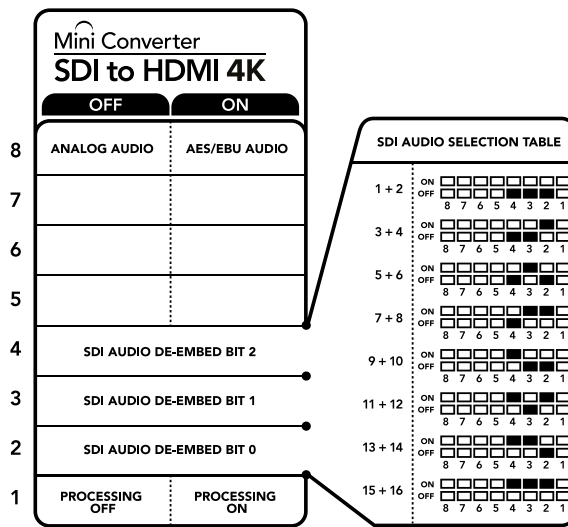
El diagrama situado en la base del convertor proporciona toda la información necesaria para modificar su configuración.
